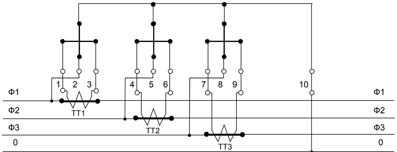
Рисунок А8. Варіант 1 - включення пряме по напрузі, трансформаторне по струму
