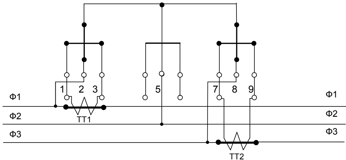
Рисунок А10. Варіант 1 - пряме включення по напрузі, трансформаторне – по струму
