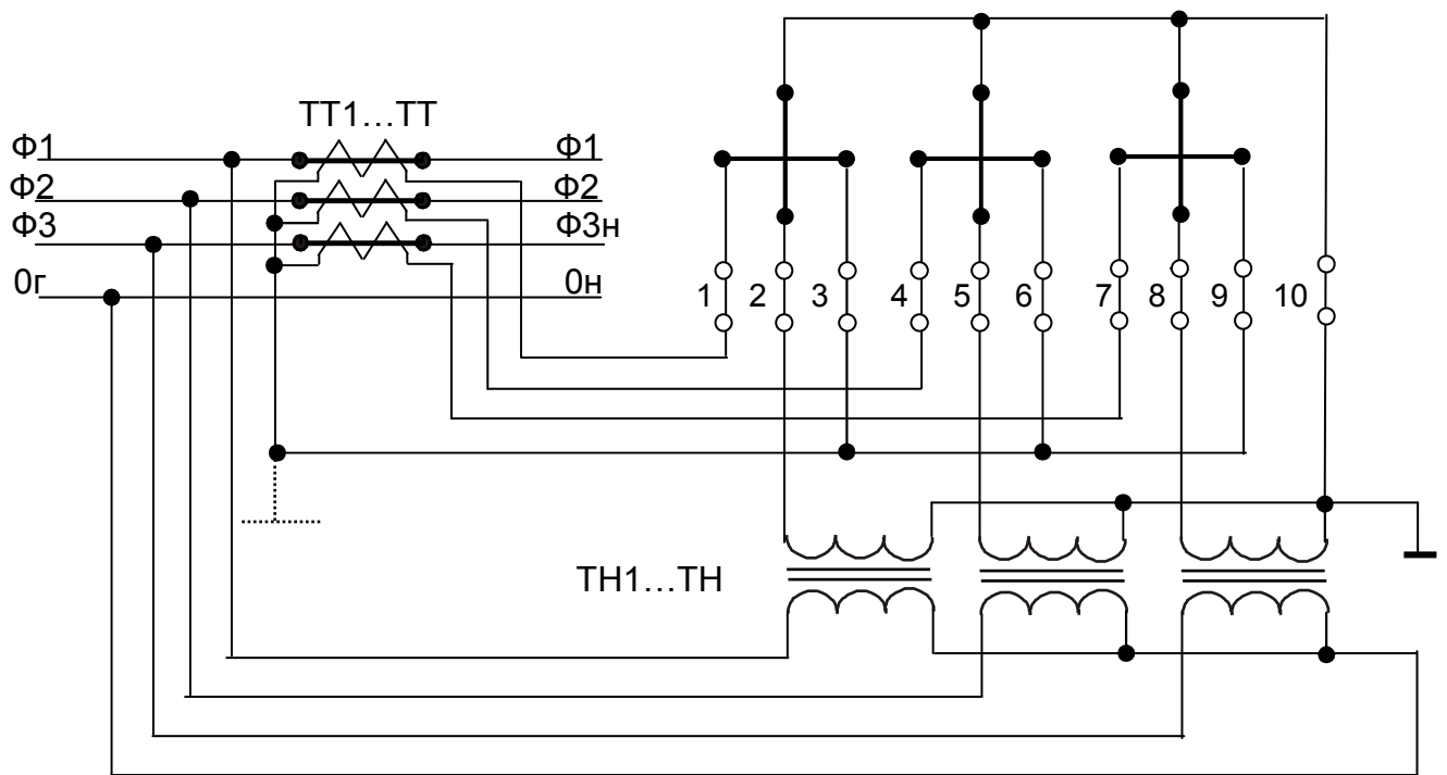
Рисунок А9. Варіант 2 - трансформаторне включення по напрузі та струму
