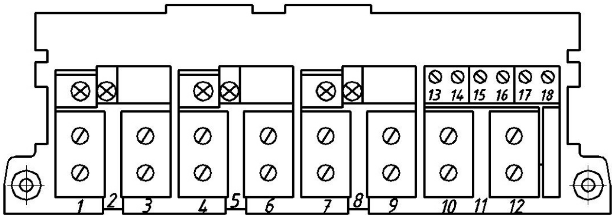
Рисунок А5. Призначення клем (контактів) лічильників прямого включення
