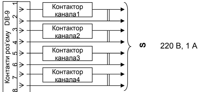
Рисунок Б1. Підключення ланцюгів управління навантаженням
