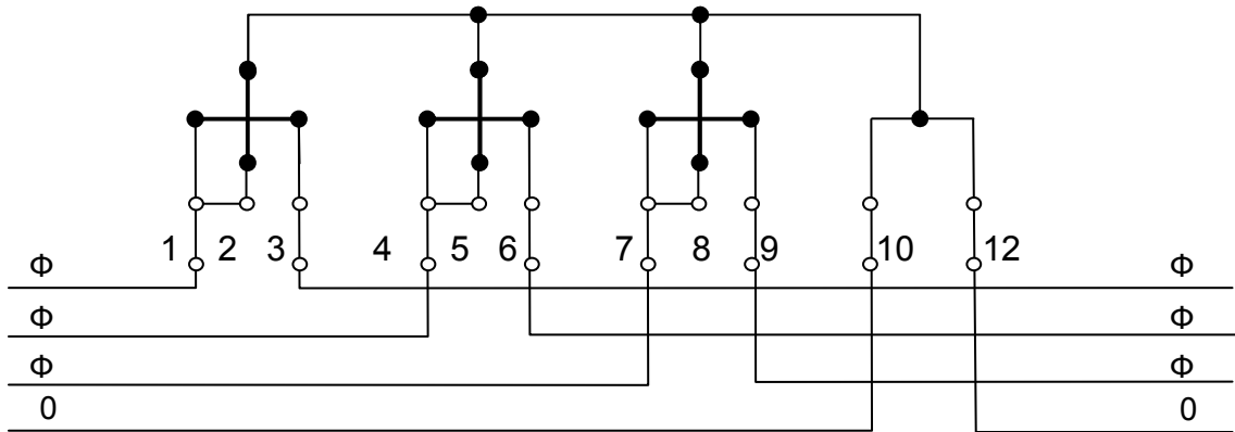
Рисунок А7. Призначення клем лічильника СТКЗ трансформаторного включення
