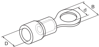
Рисунок 2. Наконечники типа НКИ
