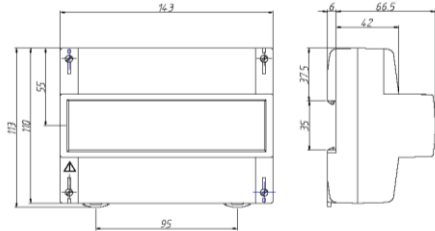
Рисунок 1 - Загальний вигляд лічильника ЦЭ6804-U у корпусі P31
