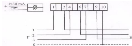
Рисунок 2 - Схема підключення лічильника
