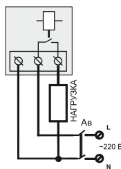
Электрическая схема
