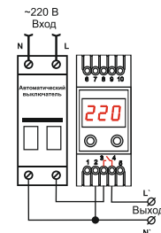
Монтажная схема
