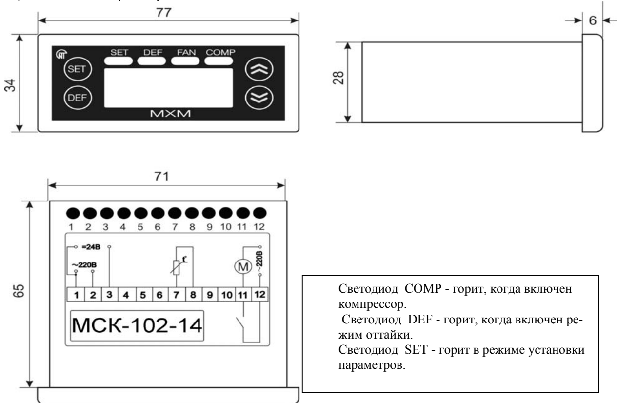
Рисунок 1. Лицевая панель, органы управления, габаритные размеры и схема подключения МСК-102-14.
